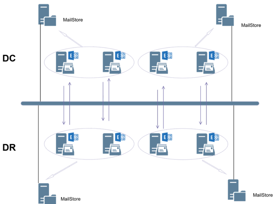
Diagrama de Implementação do MailStore
